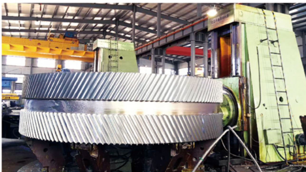
8米、14米滚齿机 直径：8m、14米 模数：40、50 8m, 14m Gear Hobbing Machine Diameter: 8m, 14m Module: 40, 50
